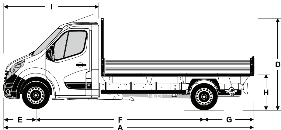
Skrzynia ładunkowa: wymiary
